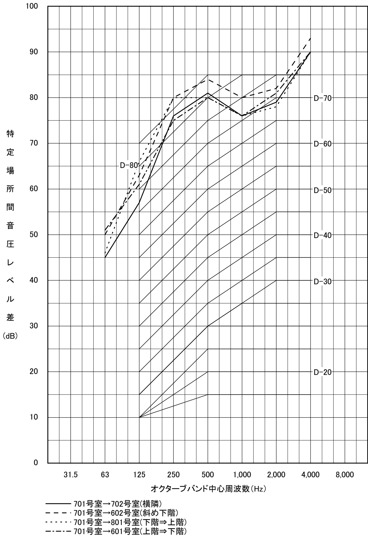
図-6 701号室→702、602、801、601号室間の遮音性能
