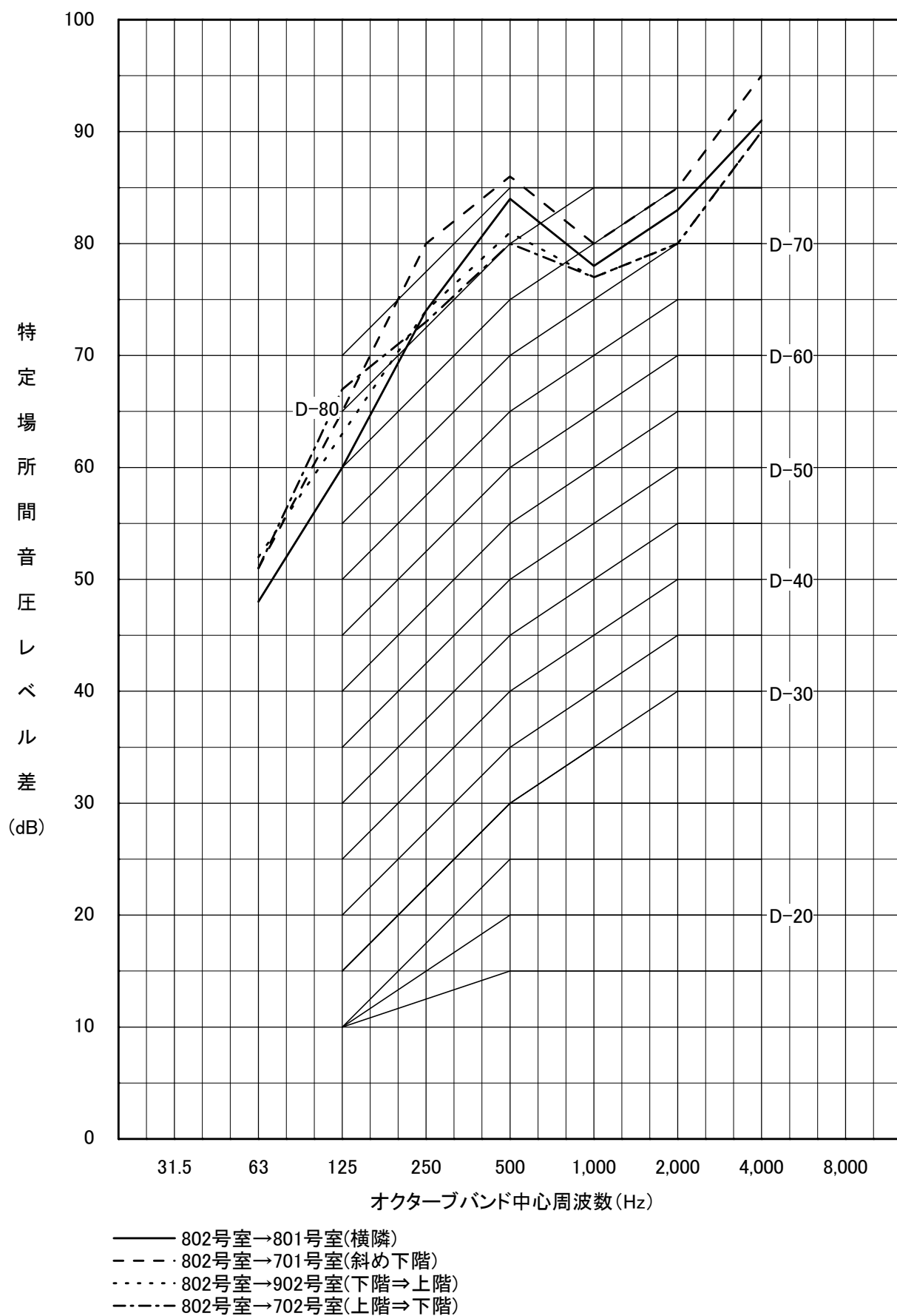
図一5 802号室→801、701、902、702号室間の遮音性能
