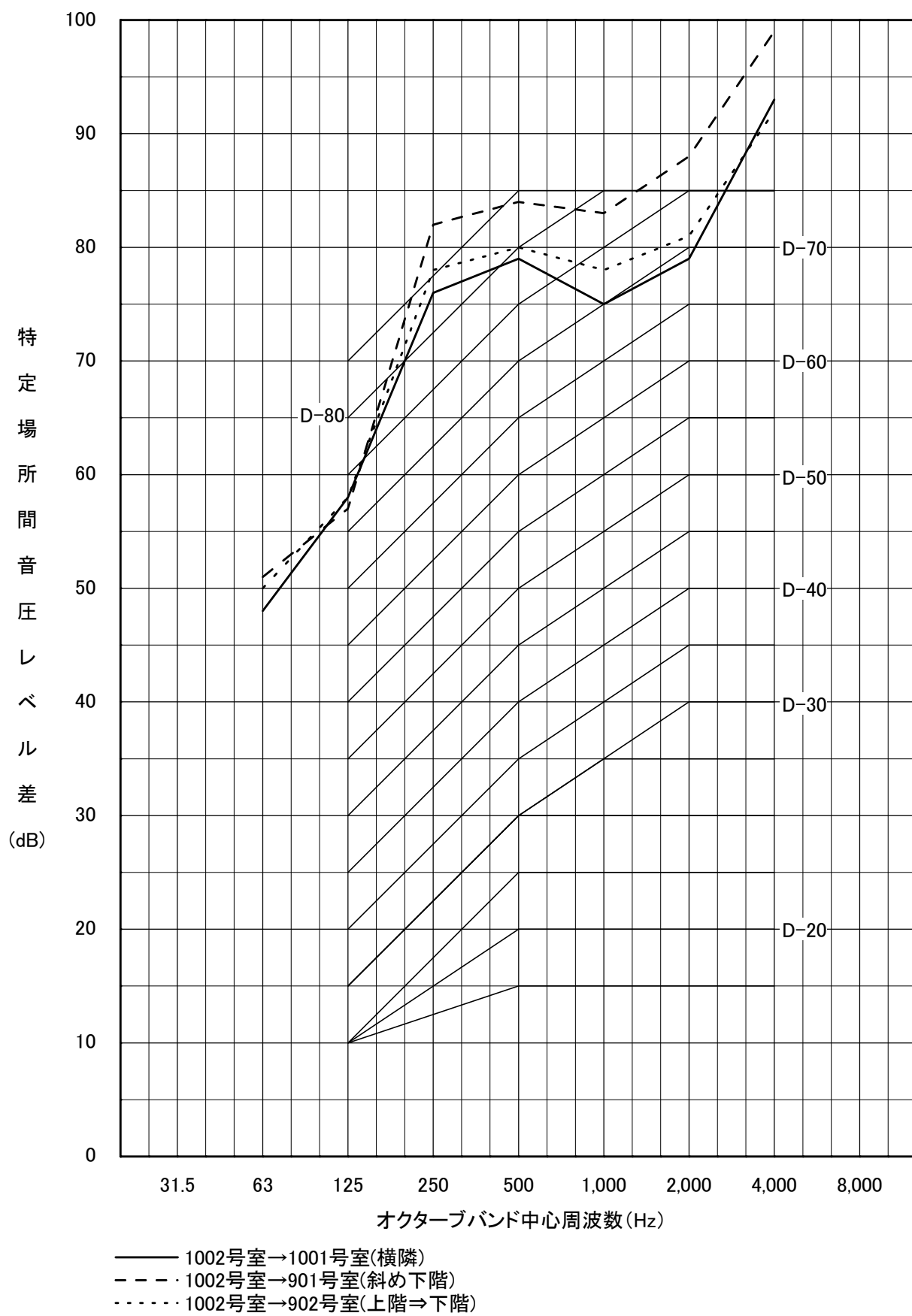
図-3 1002号室→1001、901、902号室間の遮音性能
