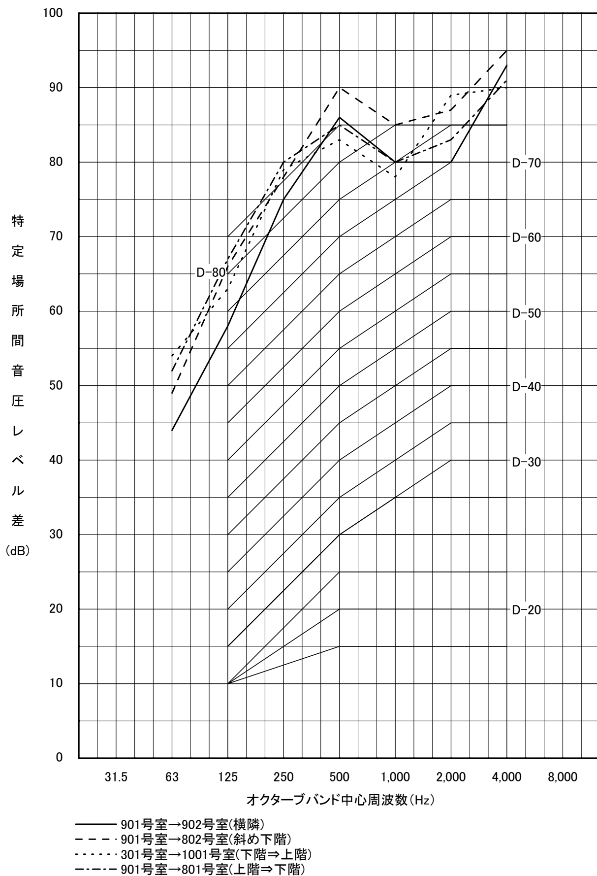
図-4 901号室→902、802、1001、801号室間の遮音性能
