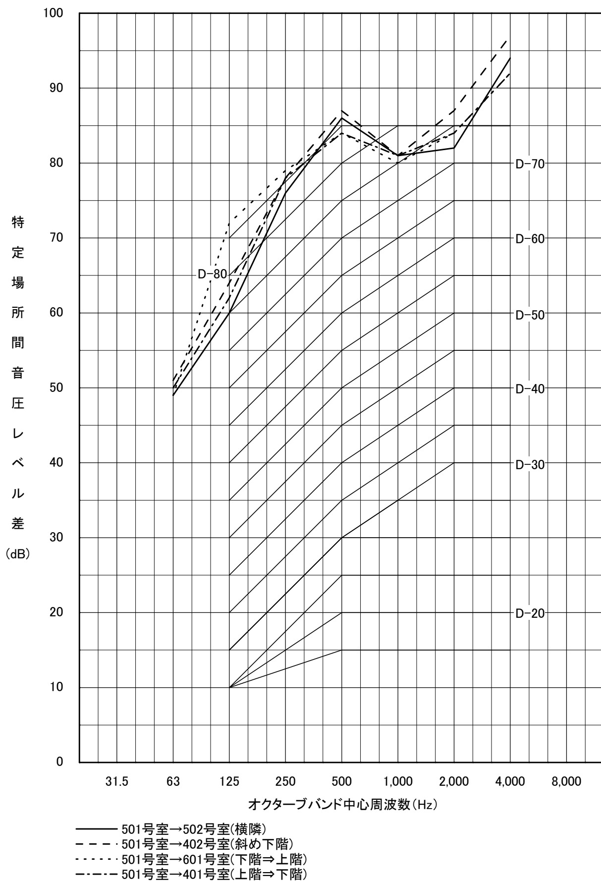
図-8 501号室→502、402、601、401号室間の遮音性能
