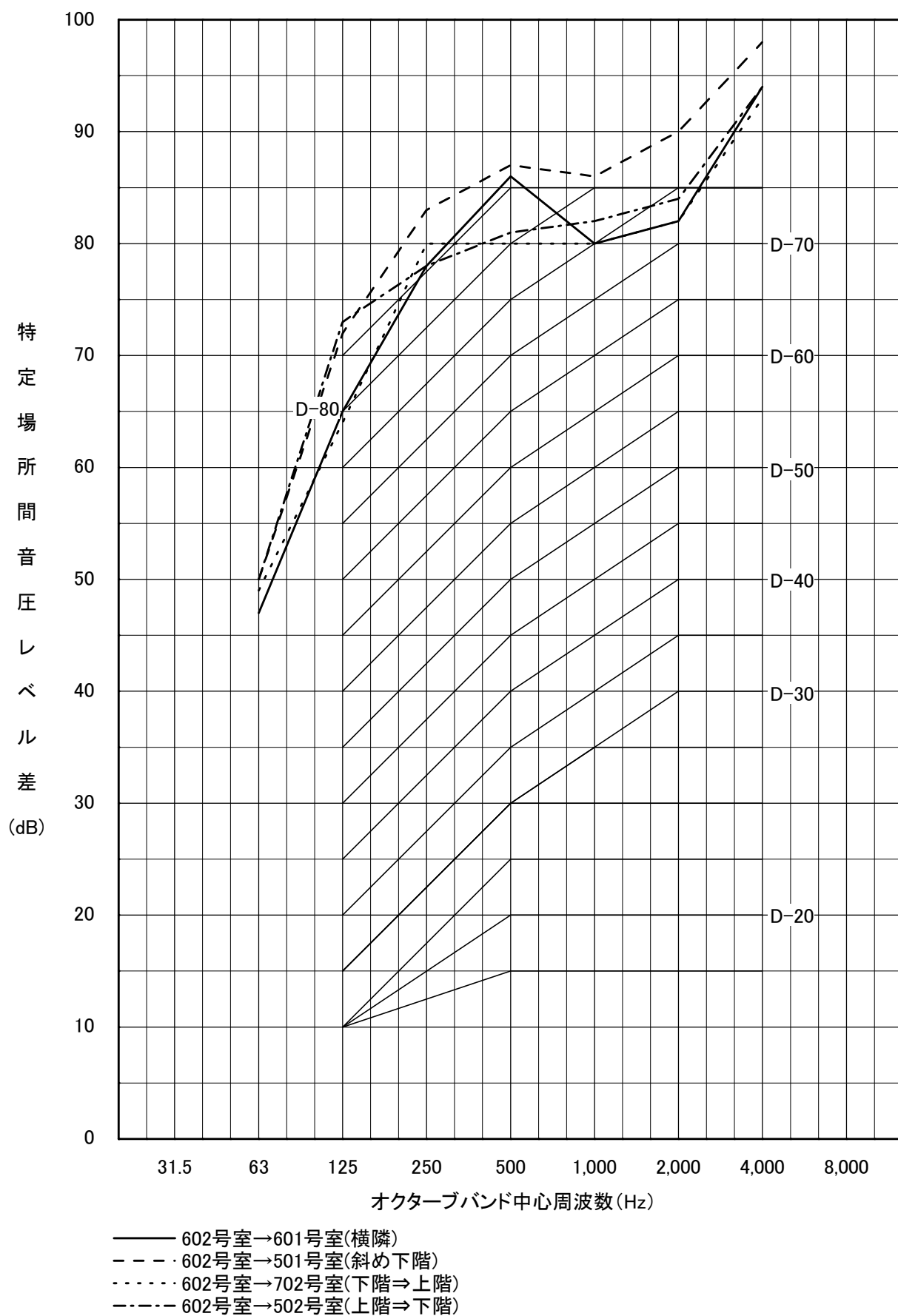
図一七 602号室→601、501、702、502号室間の遮音性能
