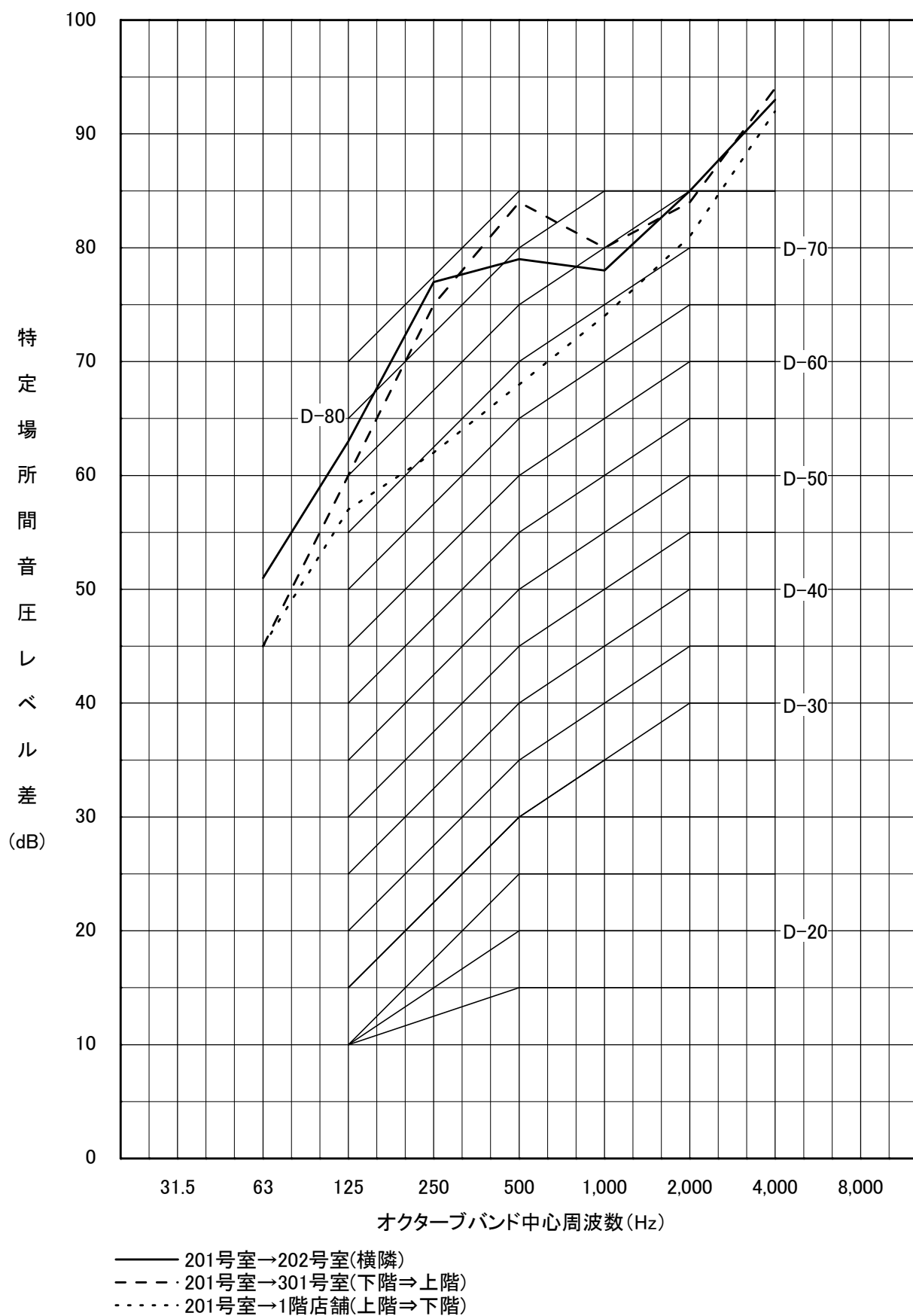
図-12 201号室→202、301号室、1階店舗間の遮音性能
