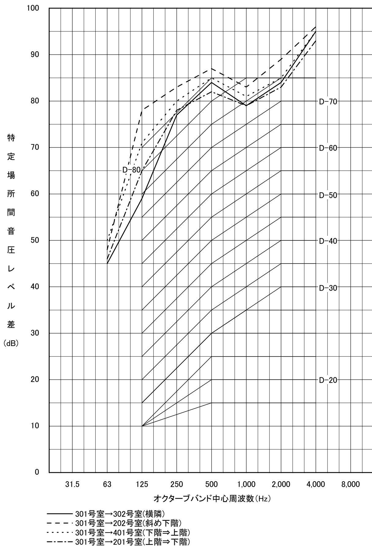
図-10 301号室→302、202、401、201号室間の遮音性能
