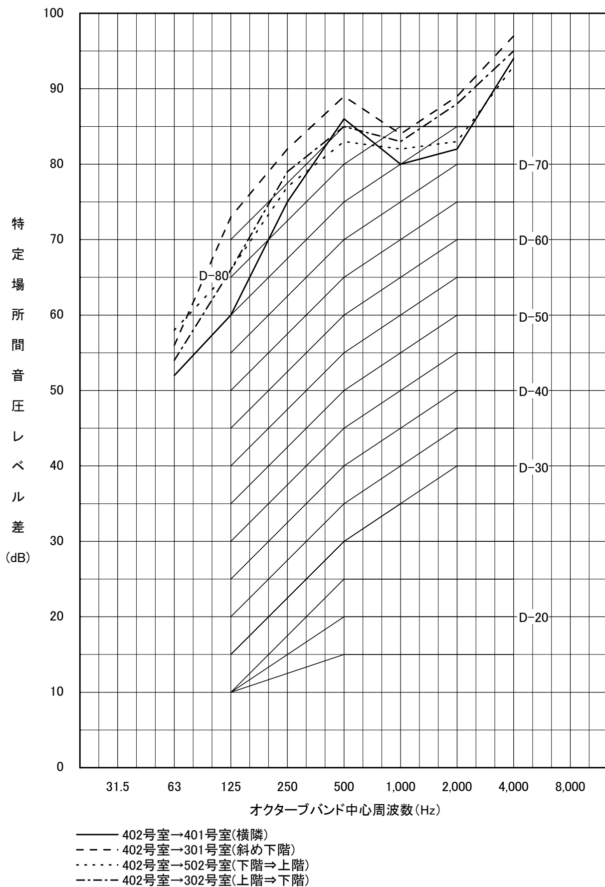
図-9 402号室→401、301、502、302号室間の遮音性能
